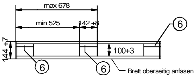
Längsansicht
