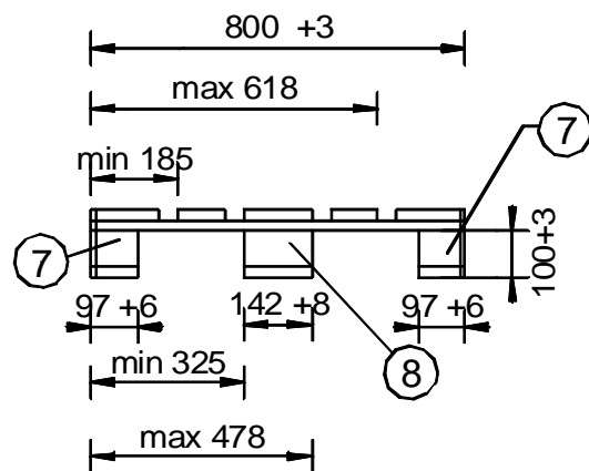
Queransicht
