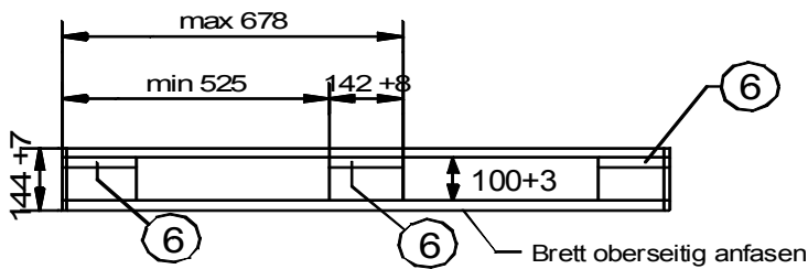
Längsansicht
